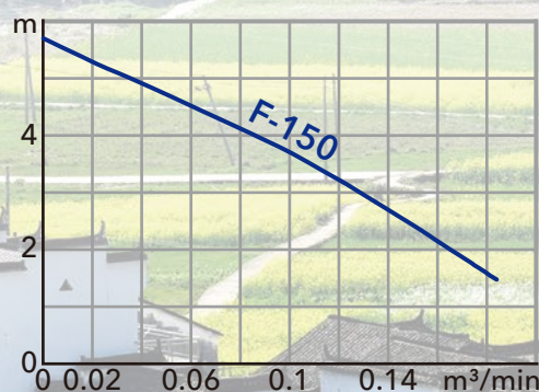
性能曲线
