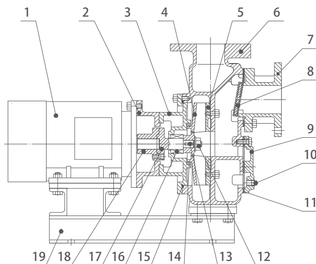
HSSD结构简图
