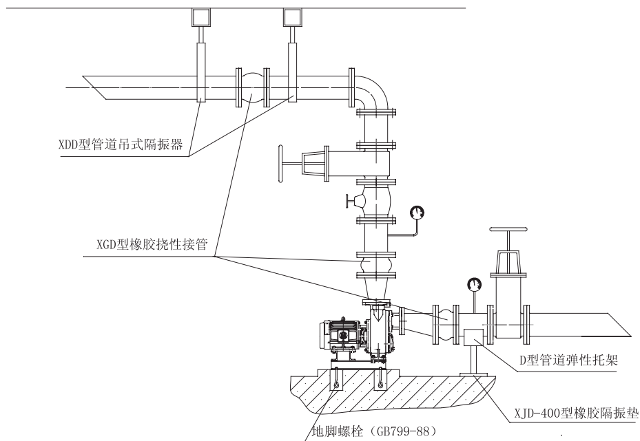
HSSD 安装示意图
